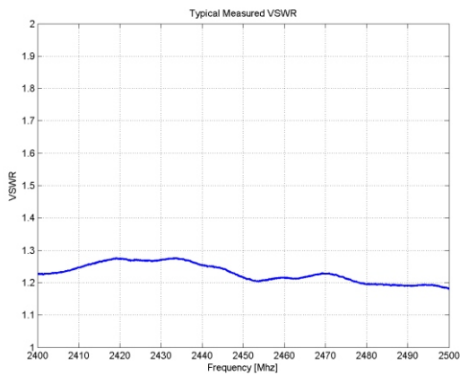
VSWR
