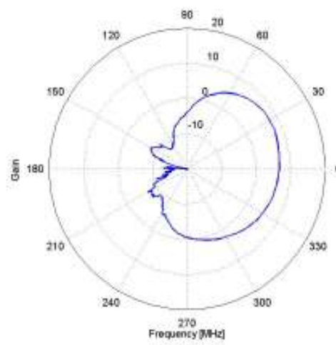
H-Plane
