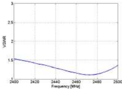
VSWR
