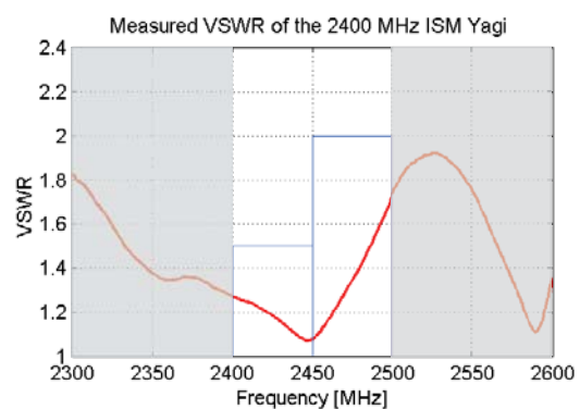
VSWR
