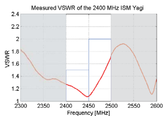
VSWR
